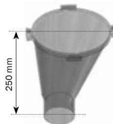
Embudo para VD5 (salida lateralizada) Artículo núm. 0221-921
