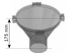
Embudo reductor VD5 (salida central) Artículo núm. 0221-939
