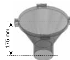
Embudo reductor VD5 (saída central) Artigo nº. 0221-939
