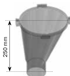
Funil para VD5 (saída lateral) Artigo nº. 0221-921
